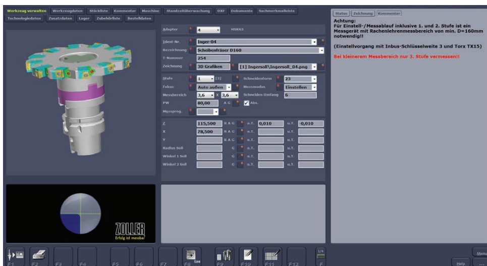
Graficzne menu obsługi »pilot 3.0«. Przejrzyste, intuicyjne menu oparte na symbolach.
