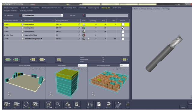
Widok magazynu narzędziowego ZOLLER »keeper« ze wskazaniem miejsca oraz z podglądem stanu magazynowego
